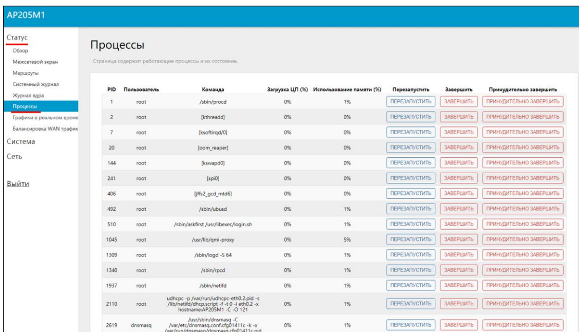
Рисунок 10.5.1 – Диспетчер процессов
