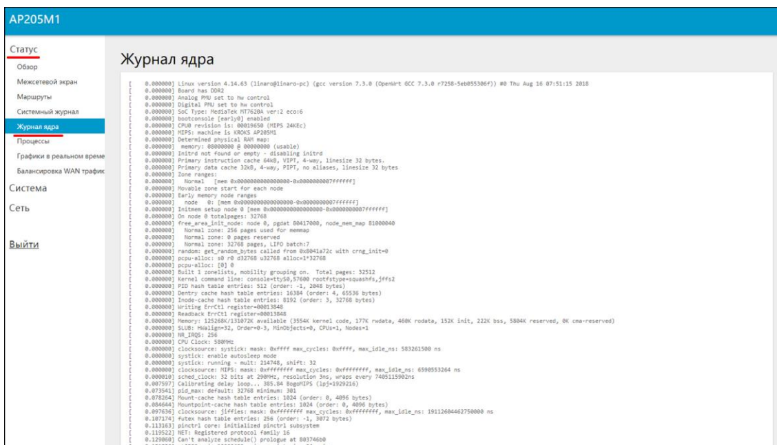
Рисунок 10.4.2 – Журнал ядра
