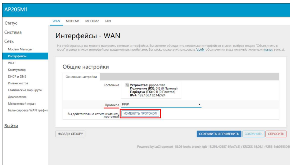
Рисунок 3.3.2 – Подтверждение выбора протокола подключения PPPtP
