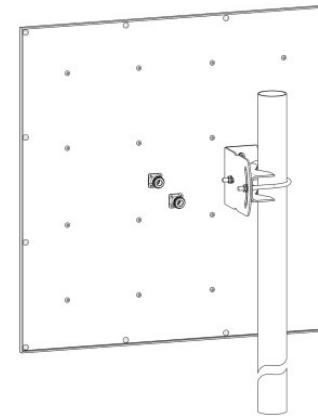
Монтаж антенны на мачте
