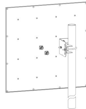
Монтаж антенны на мачте
