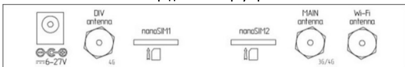
Передняя панель роутера
