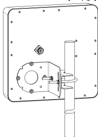
Рисунок 2 – Монтаж антенны на мачте
