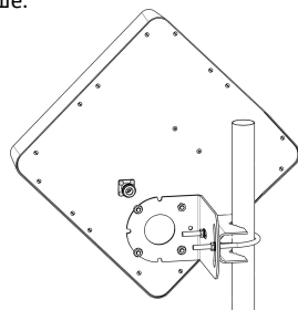
Рисунок 3 – Х-поляризация
