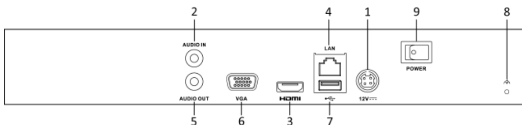
Рисунок 1.3 Задняя панель
