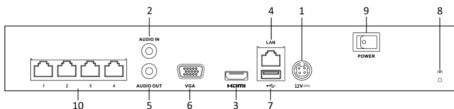
Рисунок 1.4 DS-N3XXP(B)
