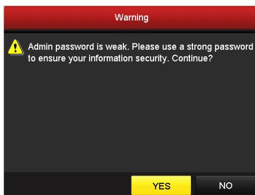
Рисунок 4.5 Окно предупреждения
